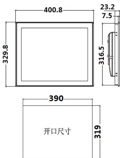
尺寸图
