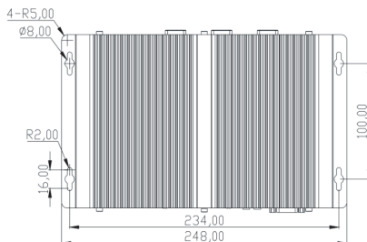
尺寸图
