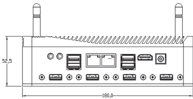
尺寸图
